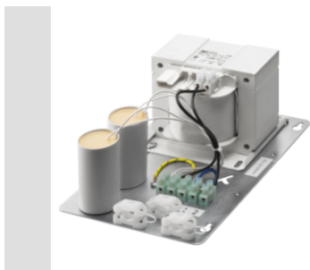
Vorschaltgeräteeinheit.
