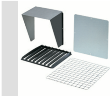
Accessorio frangiluce per HORUS 3.
