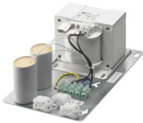
Groupe d'alimentation.
