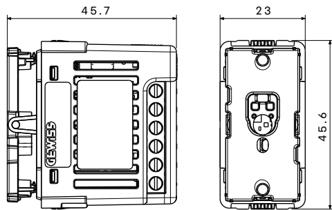
GW A1 341 Modulo di replica connesso 2 comandi
