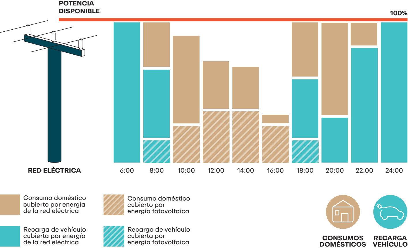
EJEMPLO DE GESTIÓN DEL CONSUMO DOMÉSTICO CON UN SISTEMA FOTOVOLTAICO
