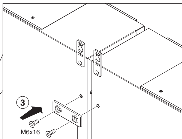
GW 47 472 (8x) Quadri a pavimento Floor panels Tableaux au sol Cuadros de suelo Schaltkästen für Bodenaufstellung
