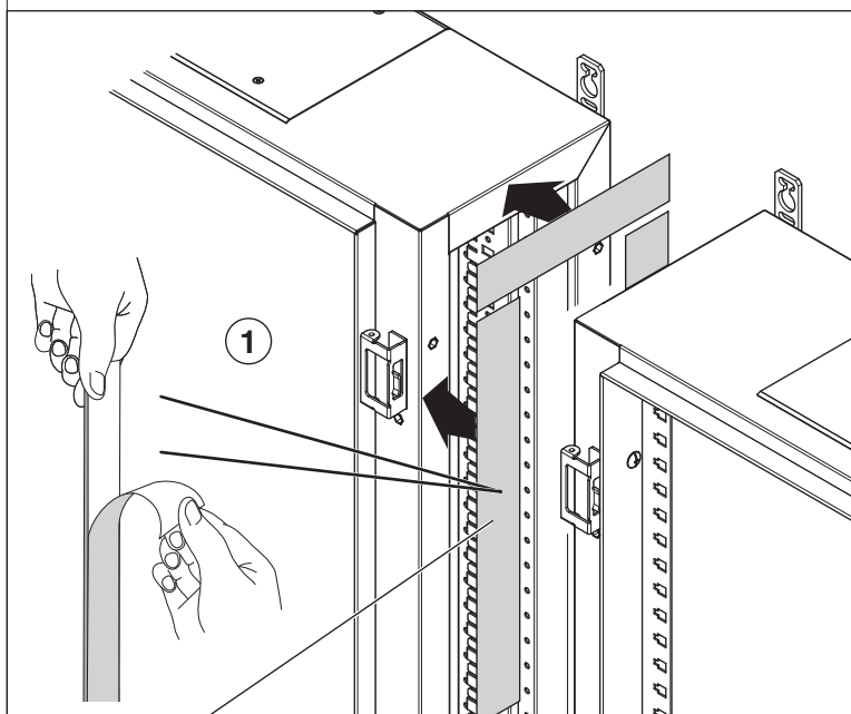
GW 47 473 Guarnizione 10x7 Seal 10x7 Garniture 10x7 Junta 10x4 Dichtung 10x7
