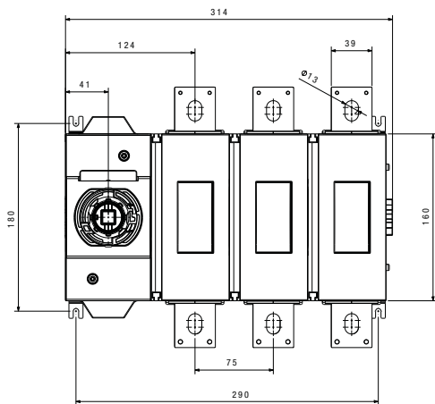
GW70091 1000A 3P
