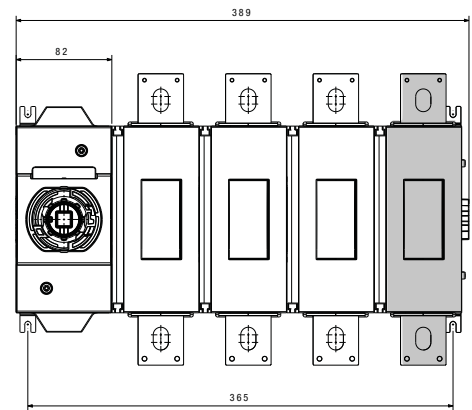
GW70092 1000A 4P
