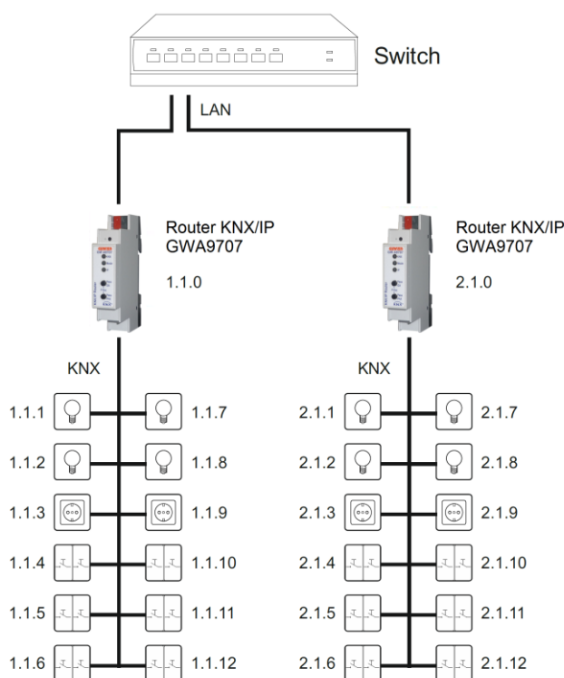
Fig 2.1: Router KNX/IP come accoppiatori di linea
