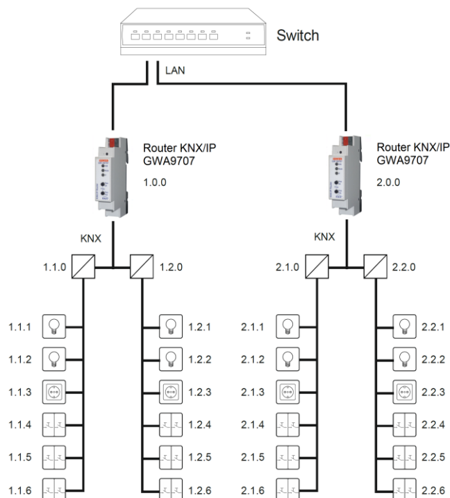
Fig 2.2: Router KNX/IP come accoppiatori di area
