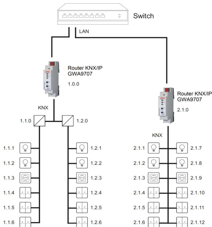
Fig 2.3: Router KNX/IP come accoppiatore di area e accoppiatore di linea
