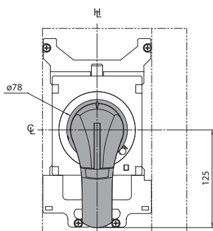
Foratura portella
