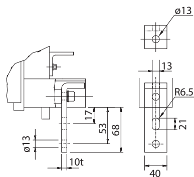
Dettaglio del collegamento Per accesso anteriore
