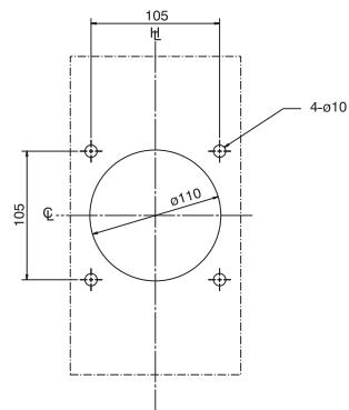
Foratura portella
