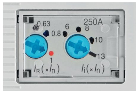
Trimmer di regolazione della corrente nominale
