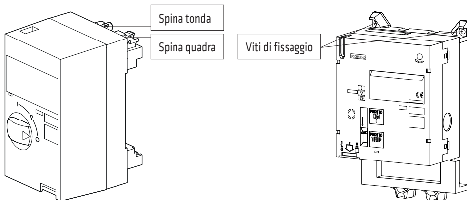
Comandi motore per interruttori taglia da 125A a 250A
