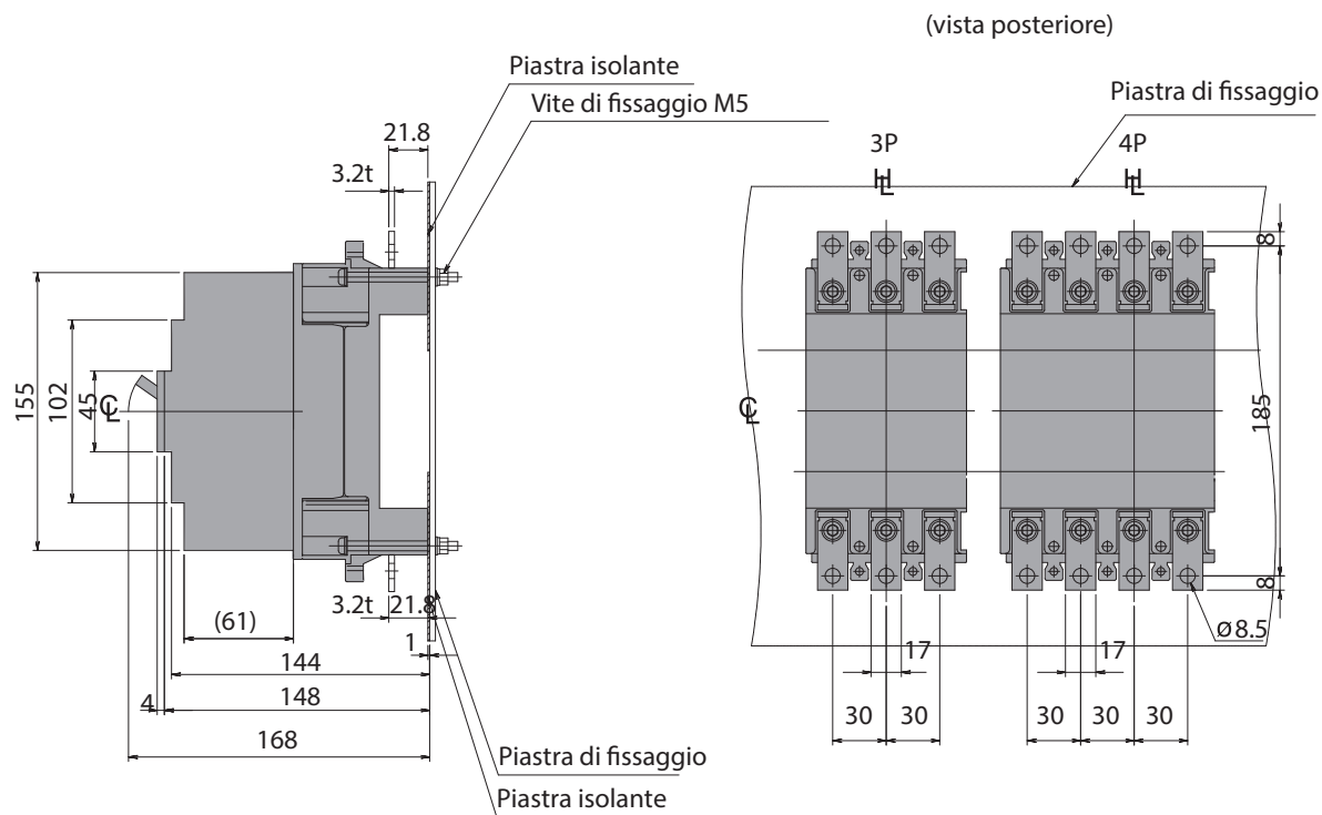
Foratura per il fissaggio (vista anteriore)
