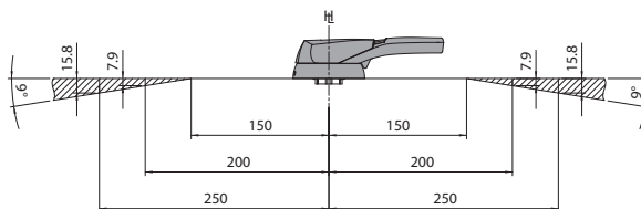
Dimensioni del lucchetto in mm (non fornito)
