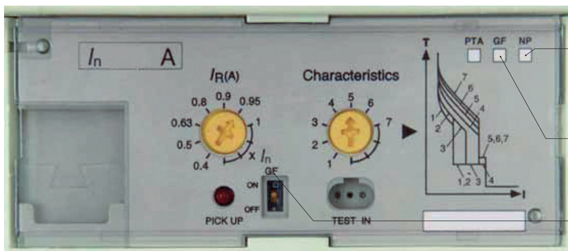
Curve protezione elettronica
