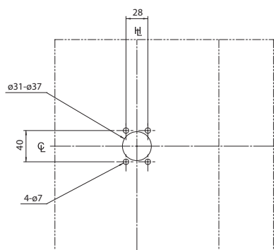
Foratura portella
