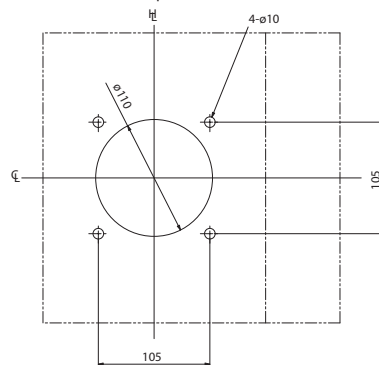
Foratura portella
