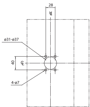
Foratura portella
