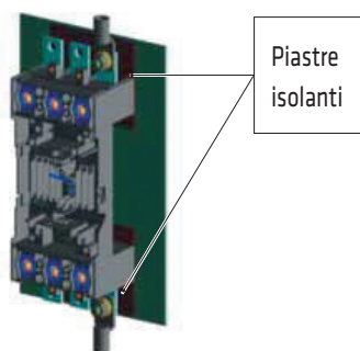
1. Base montata su piastra con terminali per accesso anteriore. Devono essere interposte piastre isolanti.
