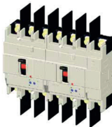
Diaframmi separatori montati tra interruttori adiacenti.
