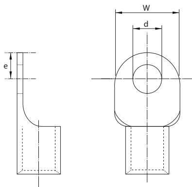
Dimensioni massime dei capicorda
