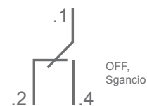
Numerazione dei morsetti
