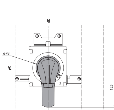
Foratura portella
