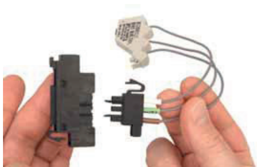
Morsettiere per un interruttore scatolato rimovibile
