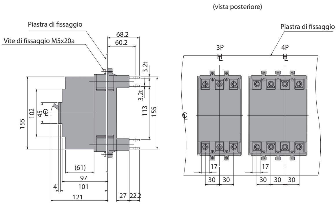
Foratura per il fissaggio (vista anteriore)
