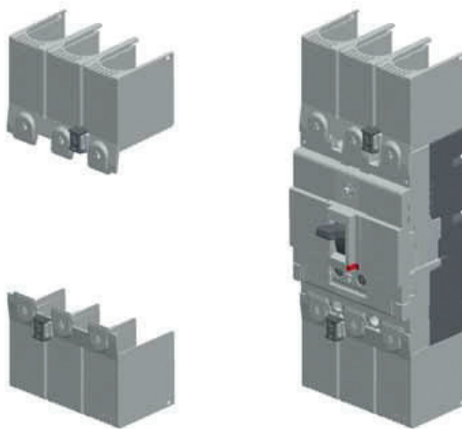
Copriterminali per terminali anteriori
