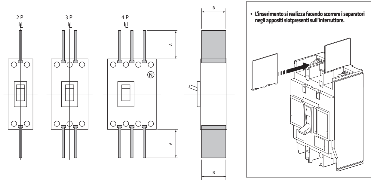
Dimensioni (mm)
