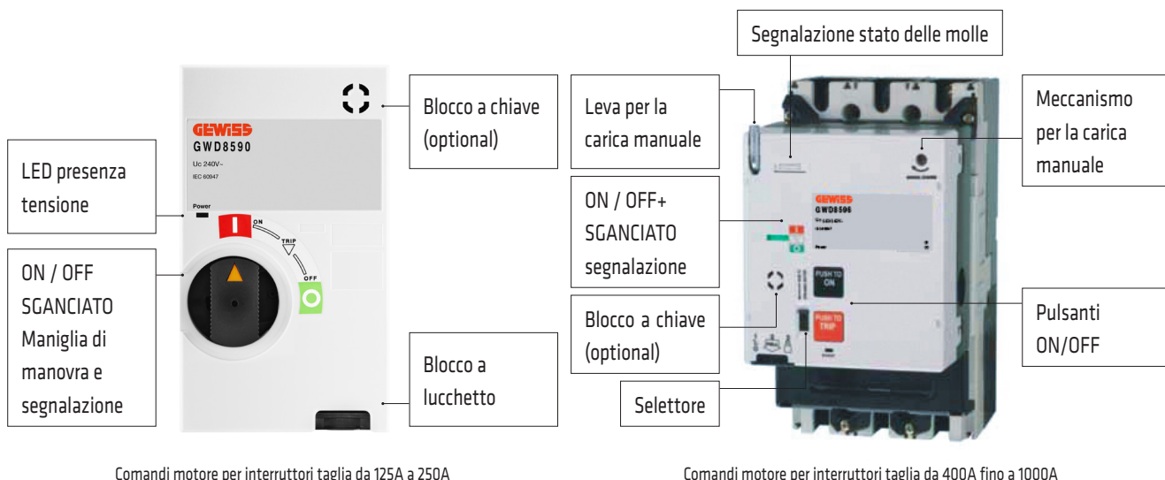
Comandi motore per interruttori taglia da 125A a 250A
