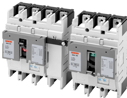
Interblocco meccanico anteriore
