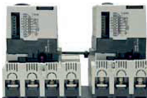
Vista dal basso dell'interblocco meccanico con comando motore
