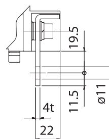
Dettaglio di collegamento per accesso anteriore
