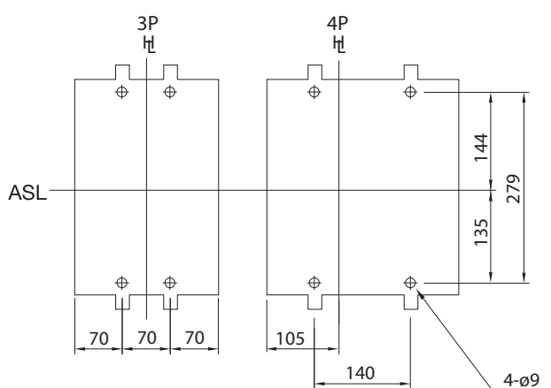
Foratura per il fissaggio (vista anteriore)
