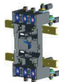
3. Base montata su profilati. Terminali predisposti per l'accessibilità posteriore.
