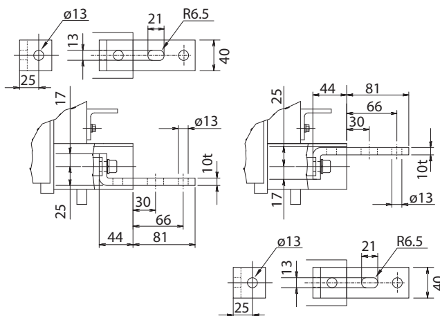
Dettaglio del collegamento Per accesso posteriore
