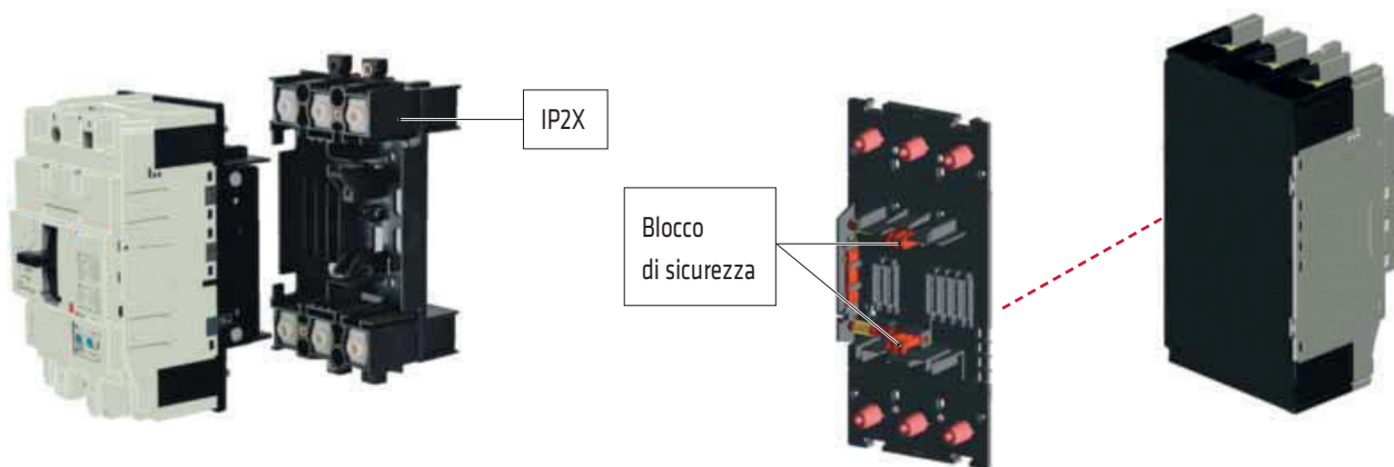
Interruttore rimovibile e base
