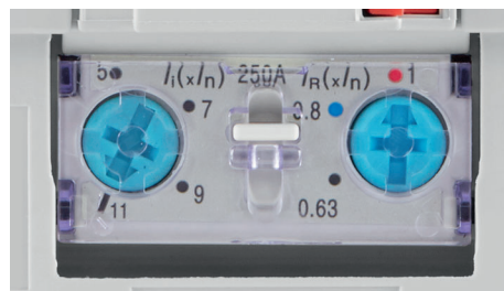
Trimmer di regolazione della corrente nominale
