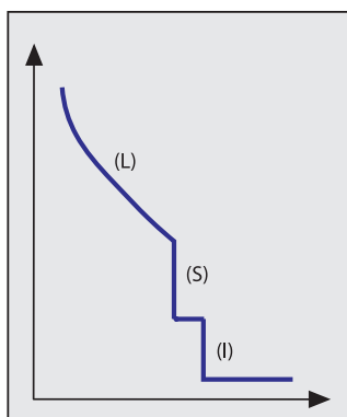
Curve protezione elettronica
