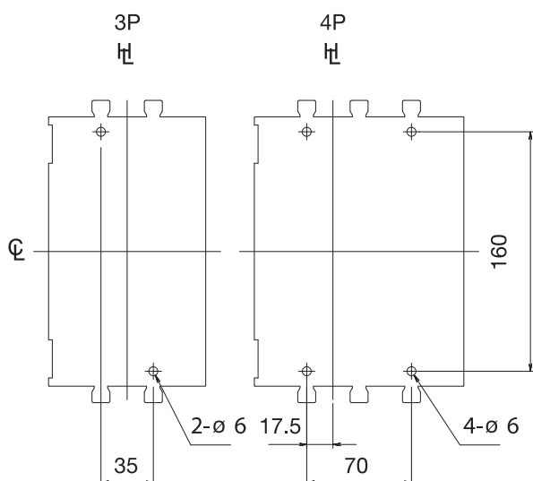
Foratura per il fissaggio (vista anteriore)
