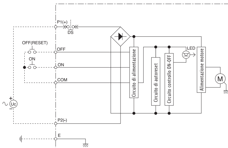
Circuito di controllo del comando motore
