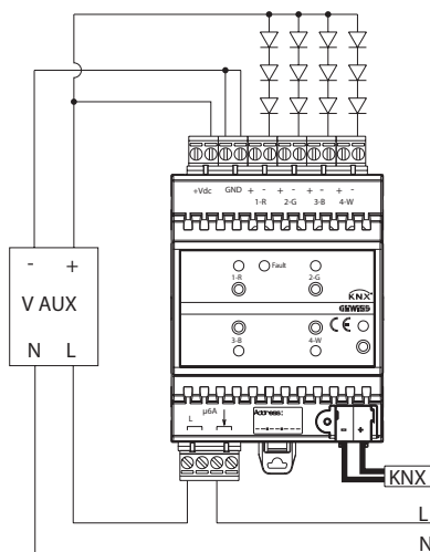
Cablaggio 2: con anodo comune connesso direttamente all'alimentazione ausiliaria LED
