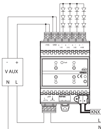
Cablaggio 1: con anodo comune connesso al dimmer
