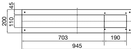
Struttura con vano affiancato
