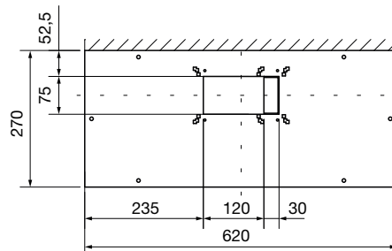
Struttura singola B=850
