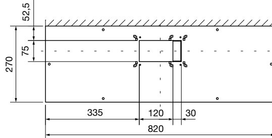
Struttura con vano affiancato
