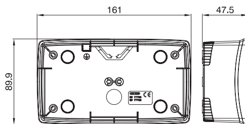
2+2 POSTI ORIZZ. GW 16 753 - GW 16 783
