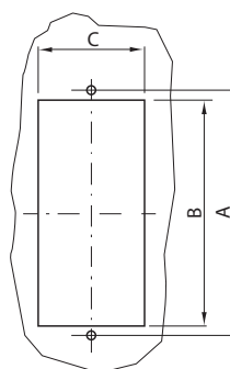
DIMENSIONI DELLO SCASSO
