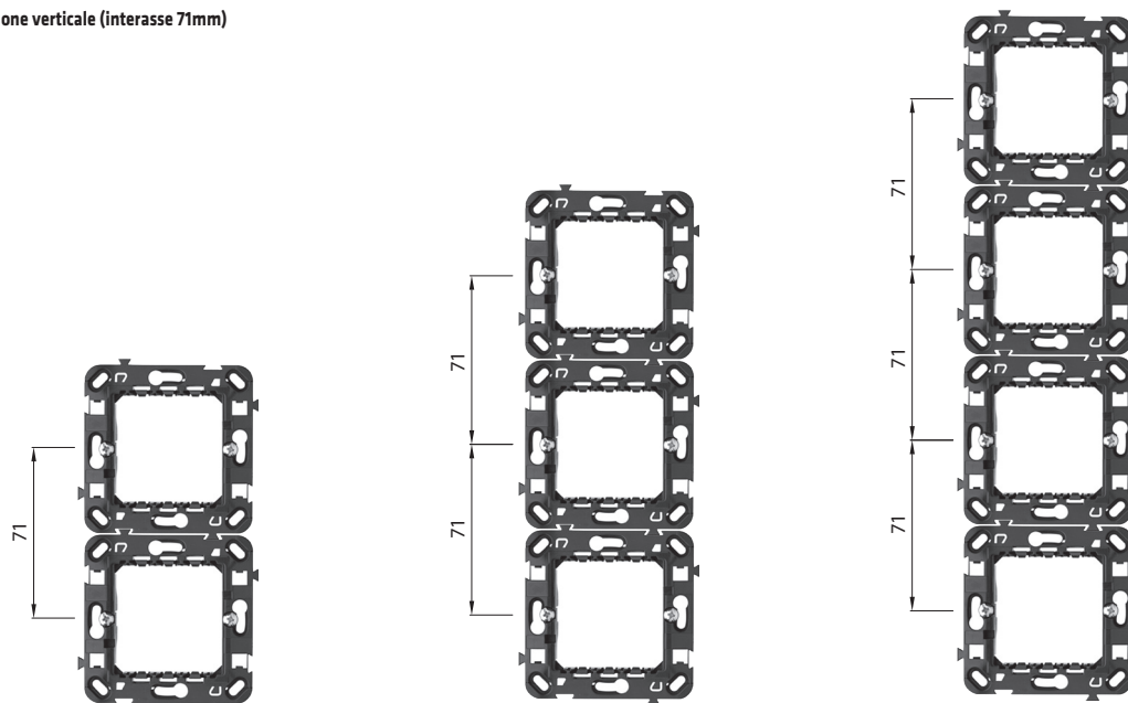
Composizione verticale (interasse 71mm)
