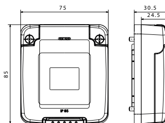
Calotta stagna con portella rigida - IP65 GW 27 403
