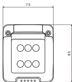
Calotta stagna con membrana - IP55 GW 27 401
